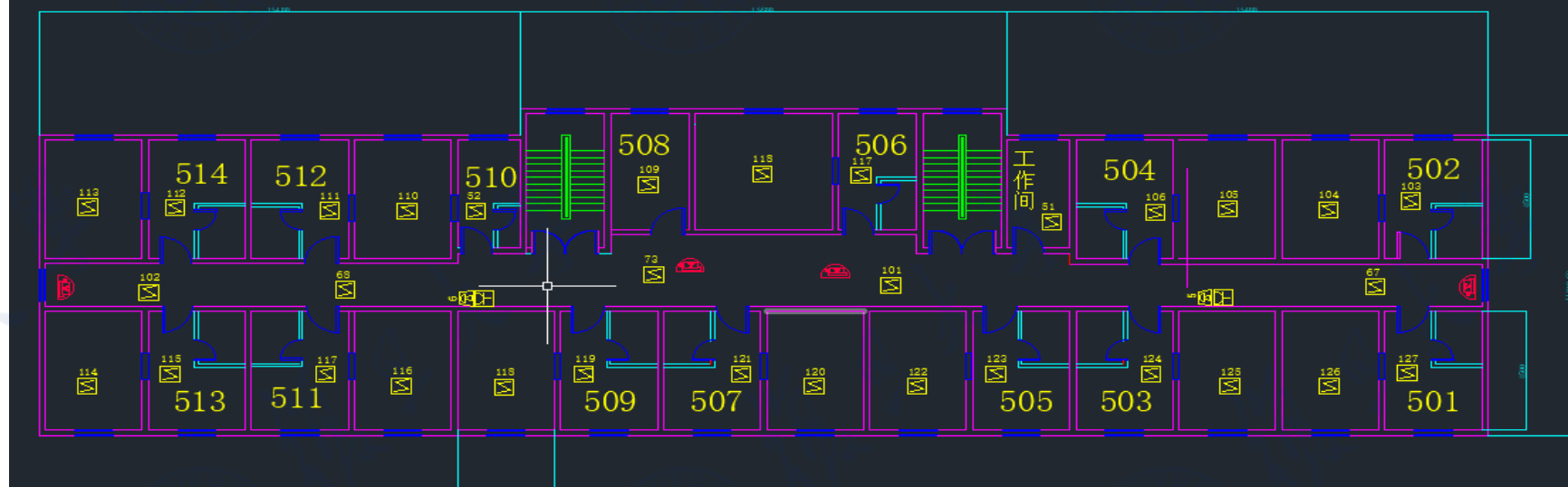
中心楼五层点位图
