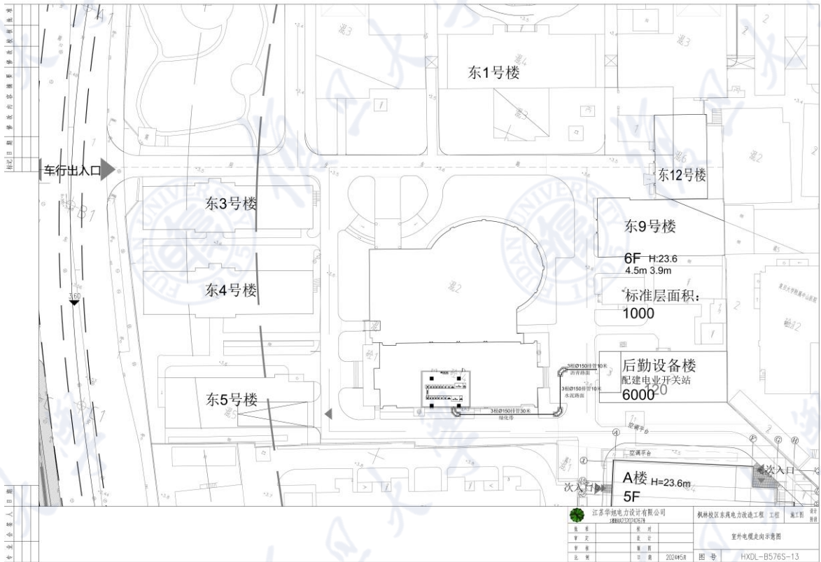
附件 A：施工现场现状平面图
